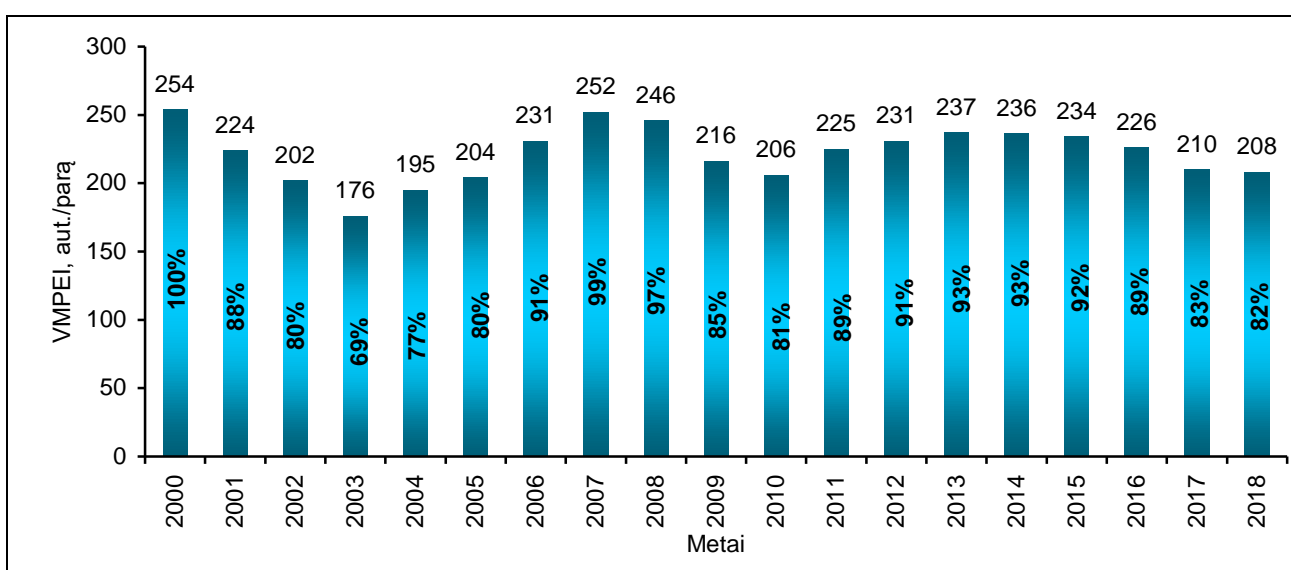
Krovinio transporto vidutinio metinio paros eismo intensyvumo kitimas krašto keliuose nuo 2000-ųjų metų
