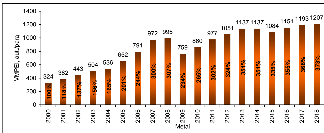
Autotraukinių (krova >12 t) vidutinio metinio paros eismo intensyvumo kitimas magistraliniuose keliuose nuo 2000-ųjų metų
