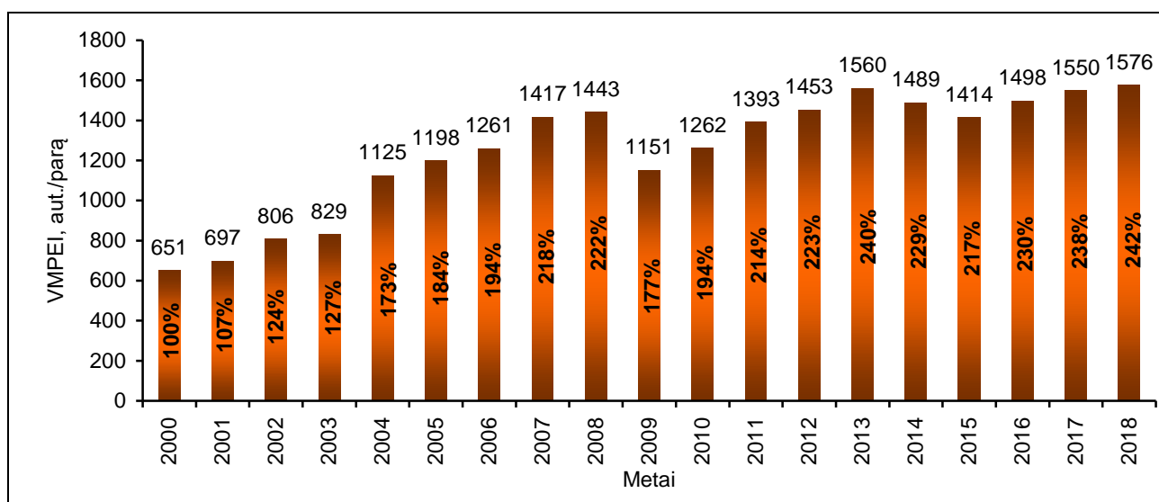
Krovininio transporto vidutinio metinio paros eismo intensyvumo kitimas magistraliniuose keliuose nuo 2000-ųjų metų
