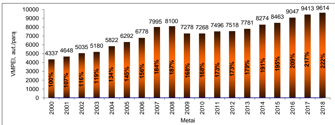
Vidutinio metinio paros eismo intensyvumo kitimas magistraliniuose keliuose nuo 2000-ųjų metų
