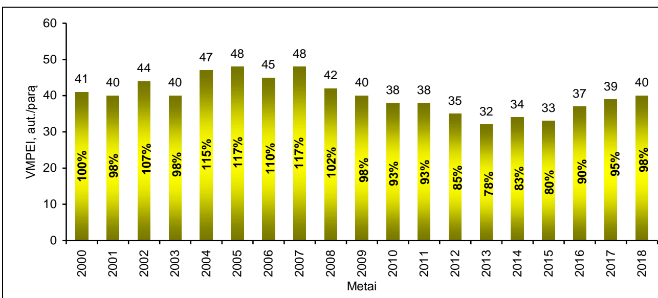
Krovininio transporto vidutinio metinio paros eismo intensyvumo kitimas rajoniniuose keliuose nuo 2000-ųjų metų
