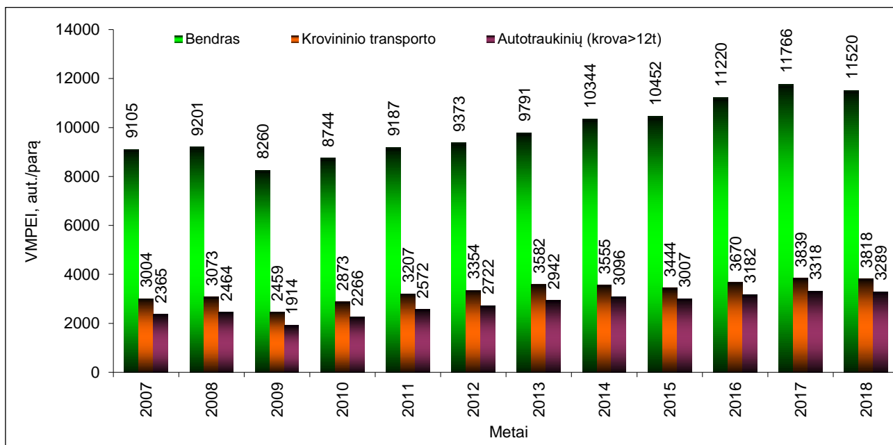
Vidutinio metinio paros eismo intensyvumo kitimas transporto koridoriuje Via Baltica nuo 2007-ųjų metų
