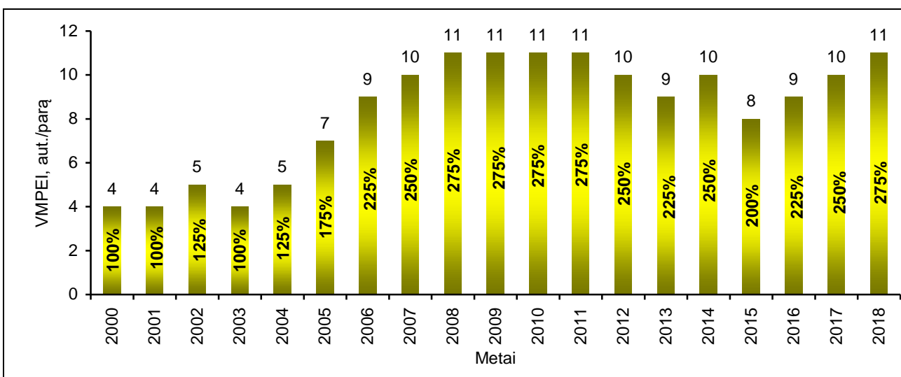
Autotraukinių (krova > 12 t) vidutinio metinio paros eismo intensyvumo kitimas rajoniniuose keliuose nuo 2000-ųjų metų
