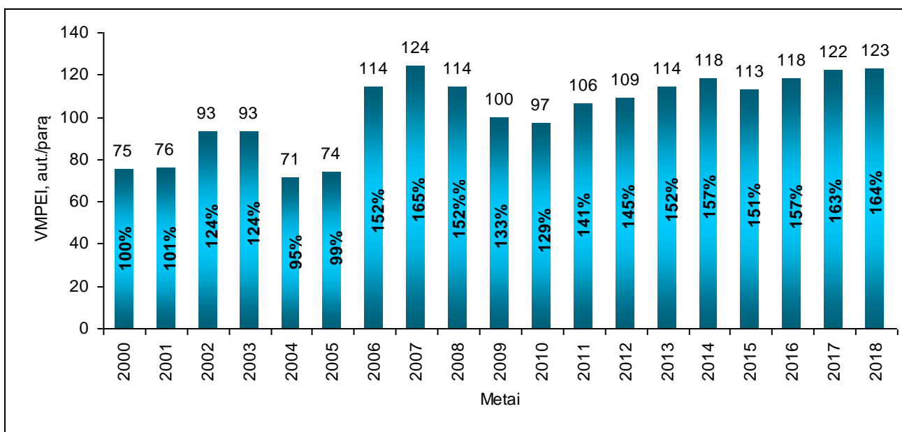
Autotraukinių (krova > 12 t) vidutinio metinio paros eismo intensyvumo kitimas krašto keliuose nuo 2000-ųjų metų
