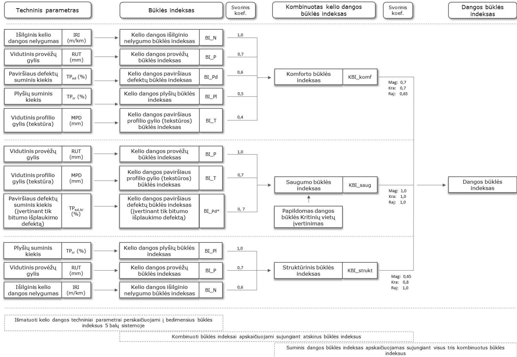
1 pav. Kelio dangos būklės vertinimo kelių tinklo lygiu struktūrinė schema
